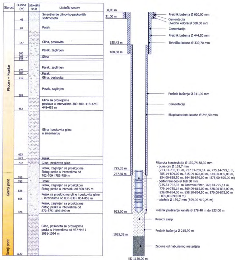
Конструкција истражно-експлоатационе хидротермалне бушотине са литостратиграфским профилем
